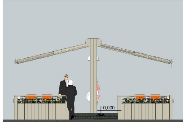
Фасад в осях А-А
